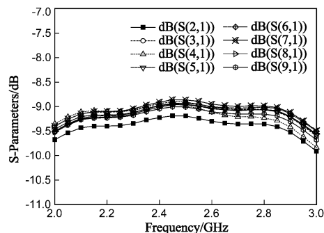
图4 功分器传输系数
