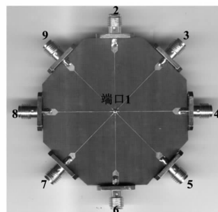
图3 9dB功分器
